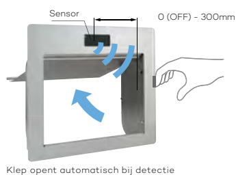
Klep opent automatisch bij detectie
